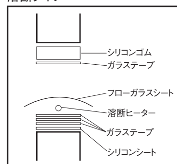
溶断タイプ
