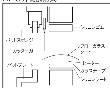
FiF-C 片側加熱式
