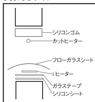
5C,10C タイプ
