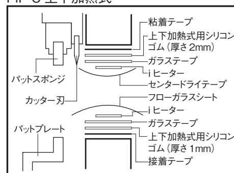
FiF-C 上下加熱式
