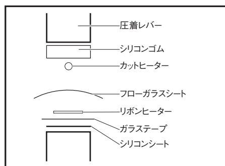
5C、10C タイプ
