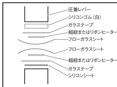
上下加熱式
