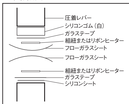
上下加熱式
