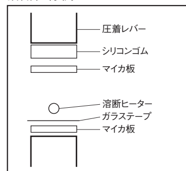
溶断仕様機
