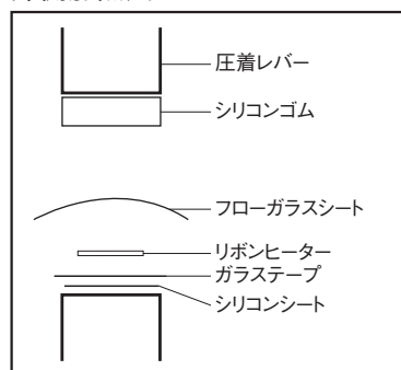
片側加熱式
