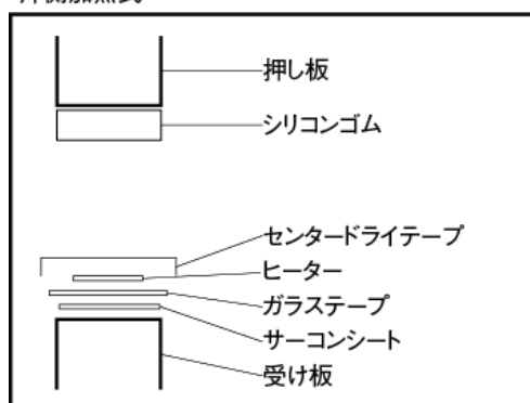
片側加熱式
