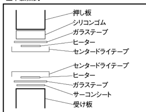
上下加熱式
