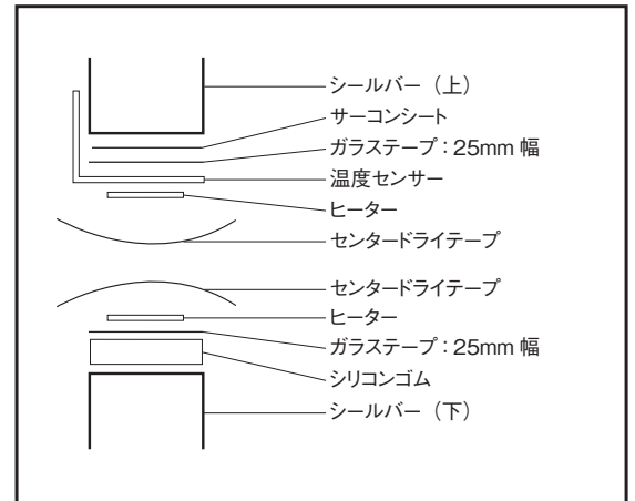
210-10W タイプ
