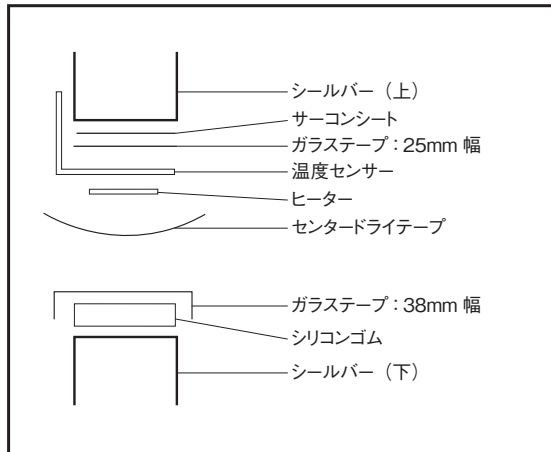
210-10、310-5、410-5 タイプ
