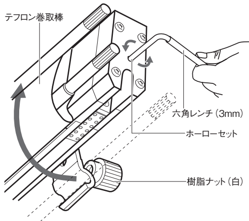
上下加熱式の圧着レバー
