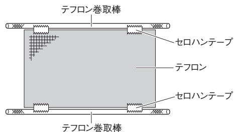
片側、上下加熱式の下部テフロン
