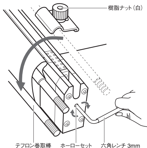
片側加熱式、上下加熱式の受け板
