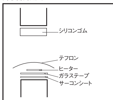
片側加熱式
