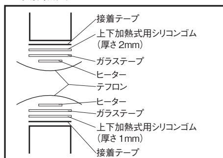
上下加熱式
