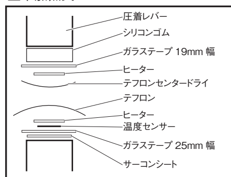
上下加熱式
