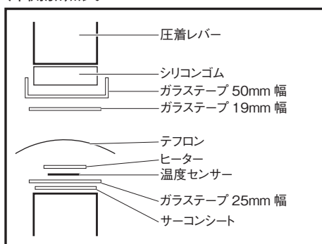
片側加熱式
