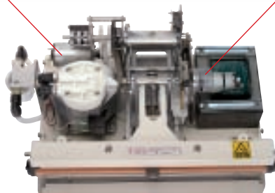
DCモーター：シール用
